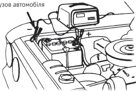
кузов автомобіля
